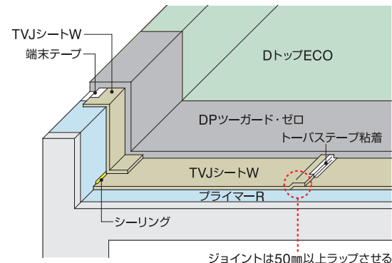
平場・立上りTVJ-W工法の場合
